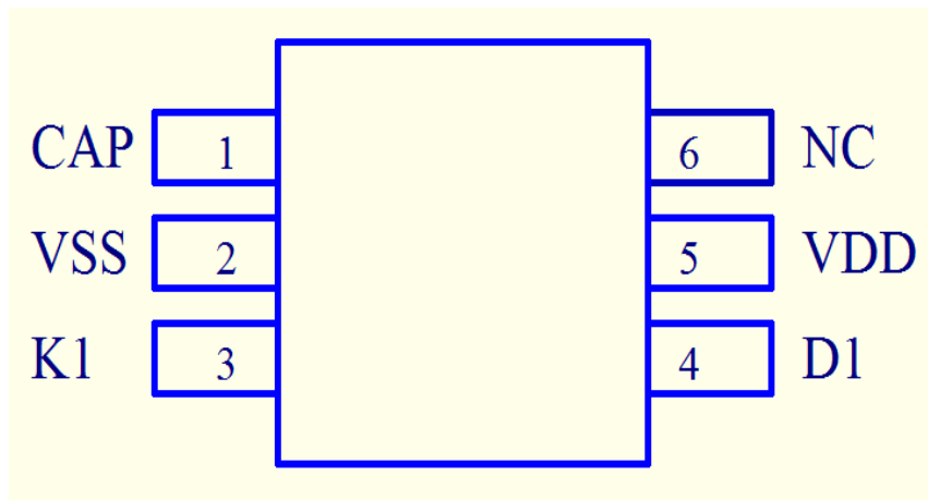
SG2301 SOT23-6-A
