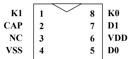
SG2908 SOP8
