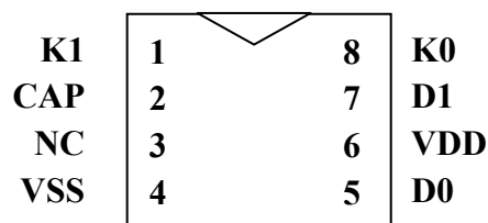
SG2938 SOP8
