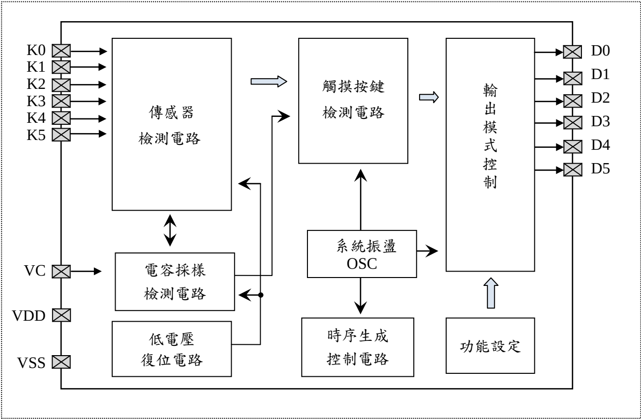
方塊圖
