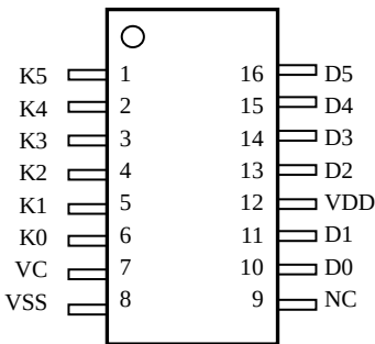
SG3256 SOP16
