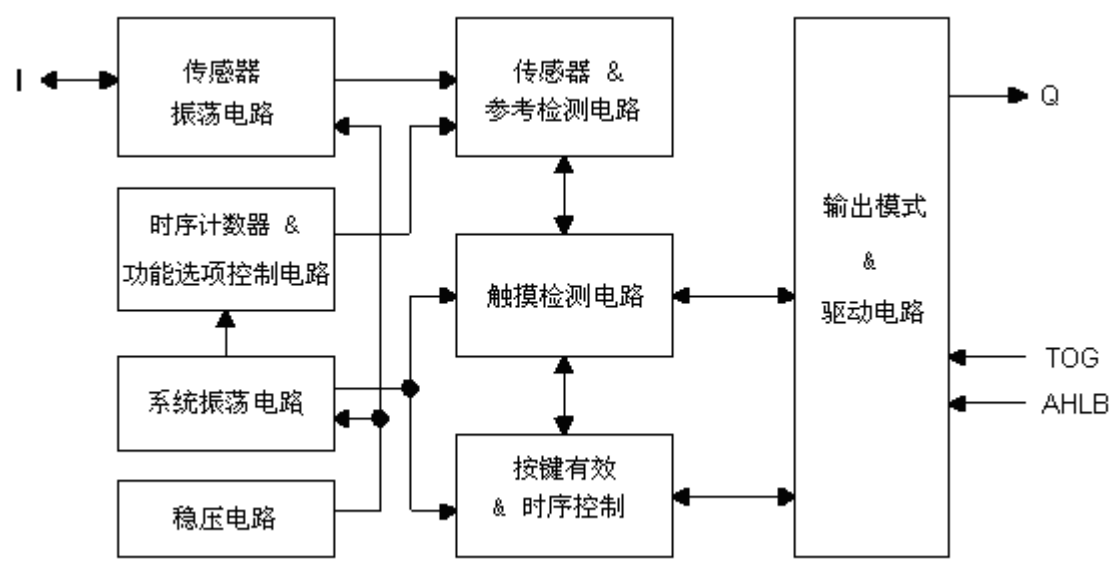
方块图
